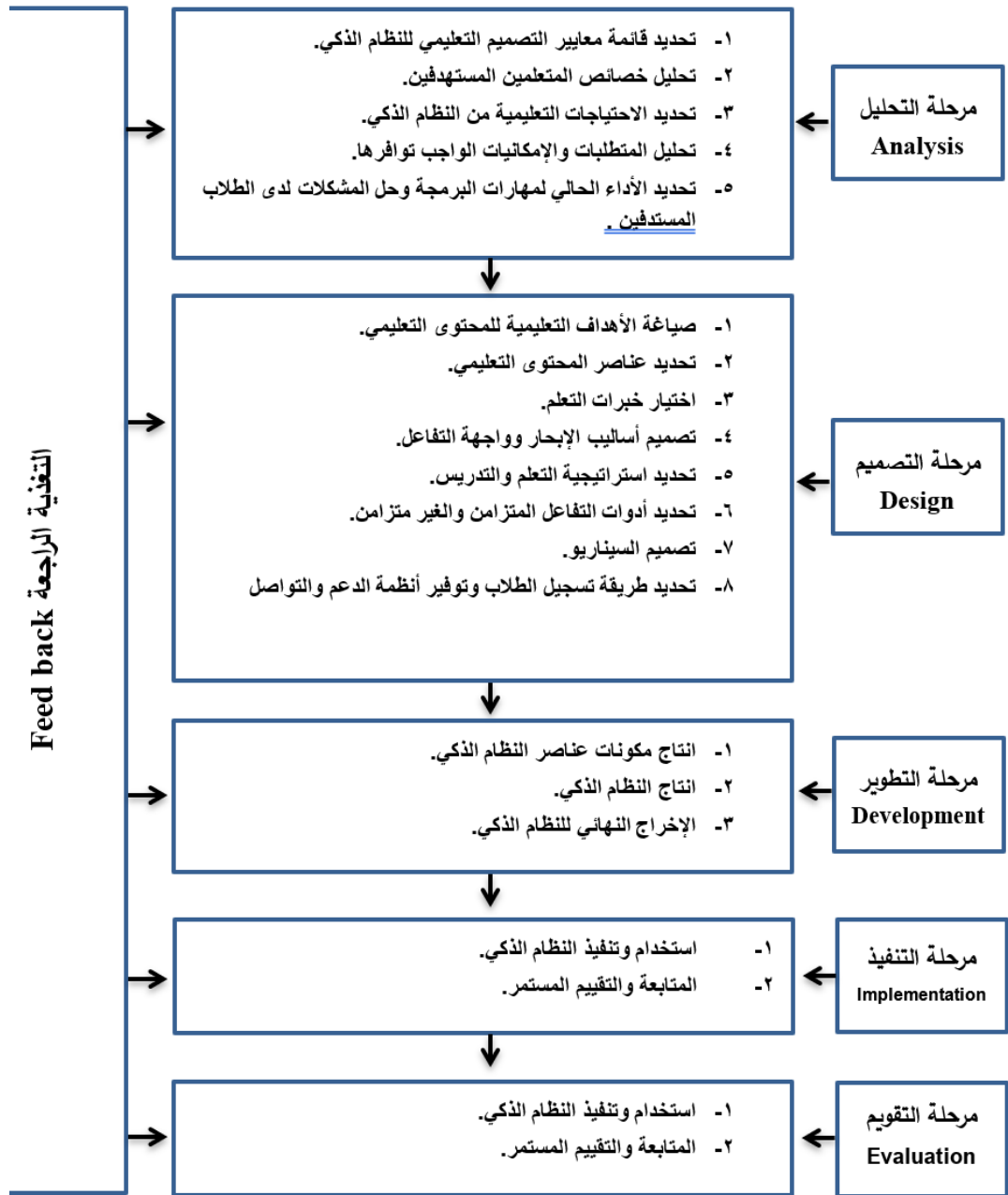
شكل (9) نموذج ADDIE (Grafinger,1988)
