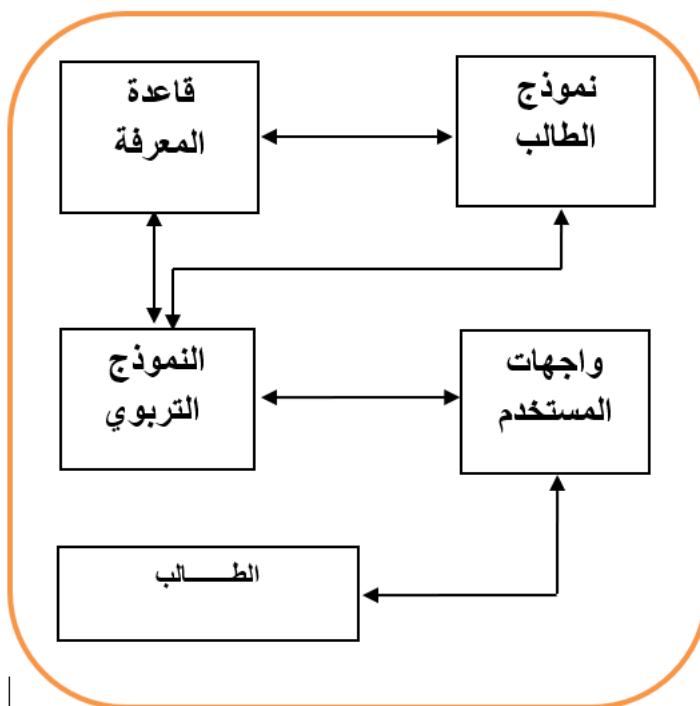
شكل (2) الوحدات المكونة لنظام التعلم الذكي
