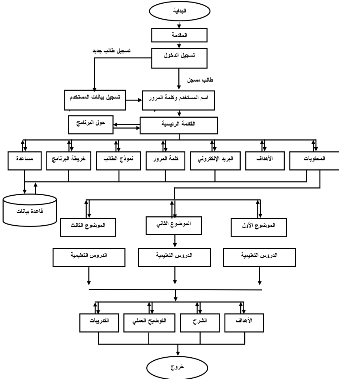
شكل (10) خريطة السير في النظام الذكي المقترح
